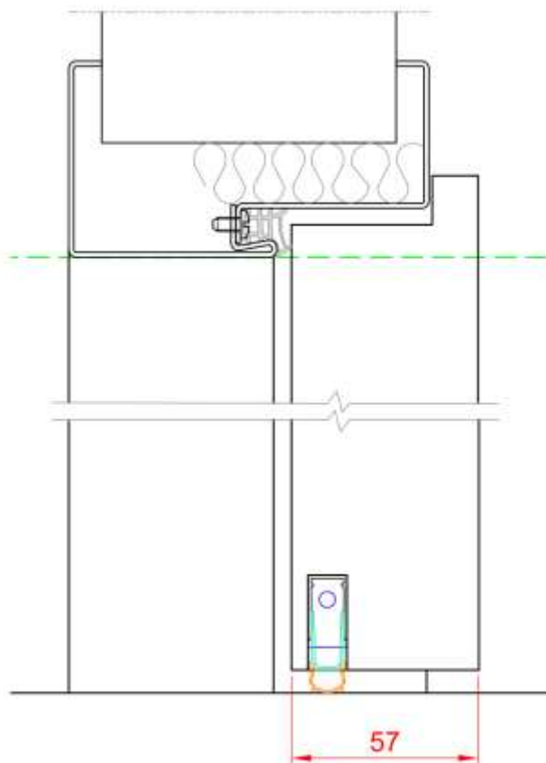
Polodrážkové dveře o tloušťce 57 mm v bezpolodrážkové zárubni
