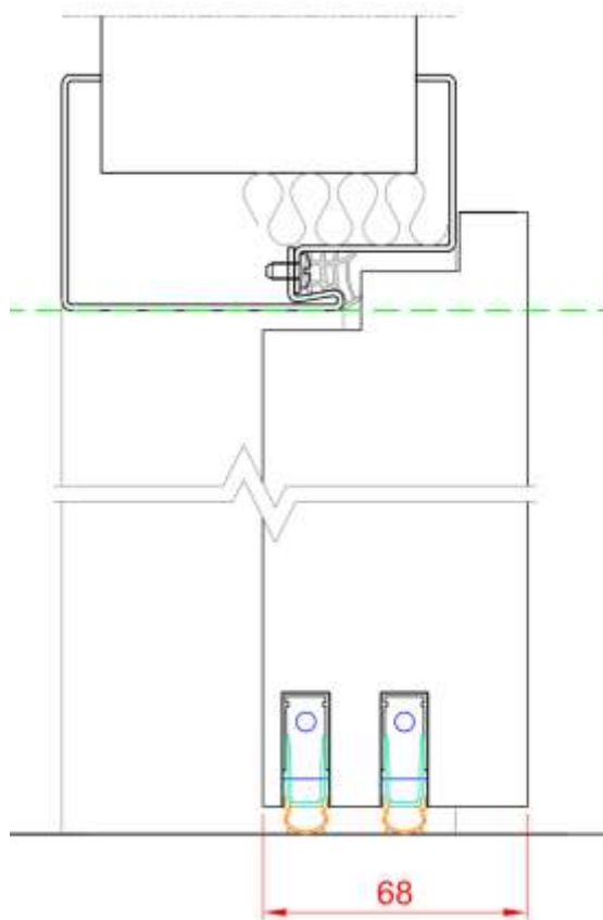
Dvoupolodrážkové dveře o tloušťce 68 mm v polodrážkové zárubni
