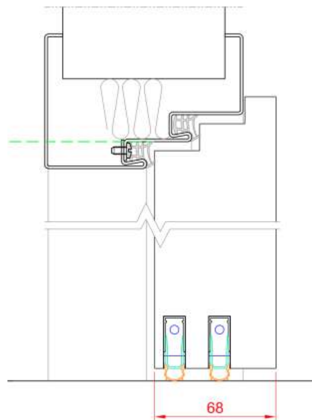
Dvoupolodrážkové dveře o tloušťce 68 mm v dvoupolodrážkové zárubni
